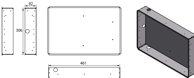
Unterputzgehäuse CP915-I, Maße in mm
