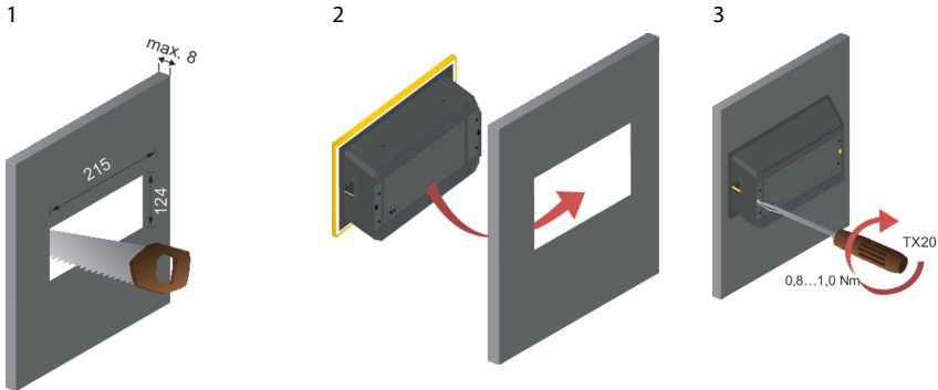
Montage in Schaltschranktür, Maße in mm
