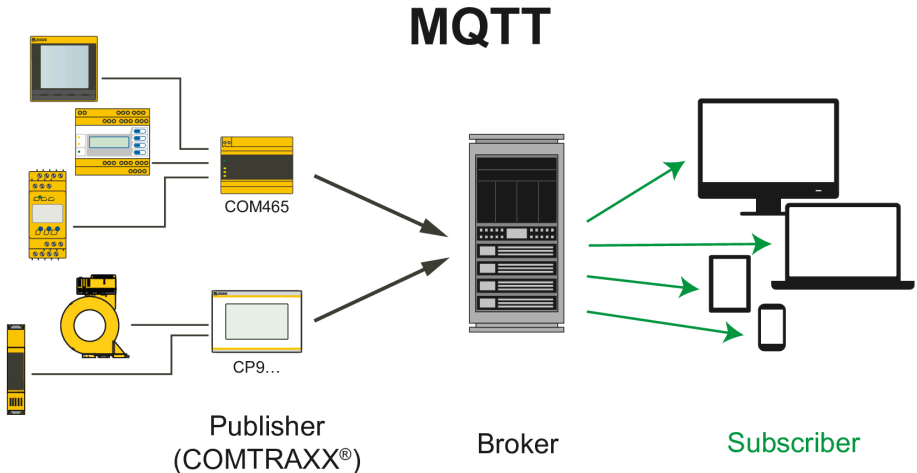
Abbildung 12-1: MQTT-Prinzipübersicht
