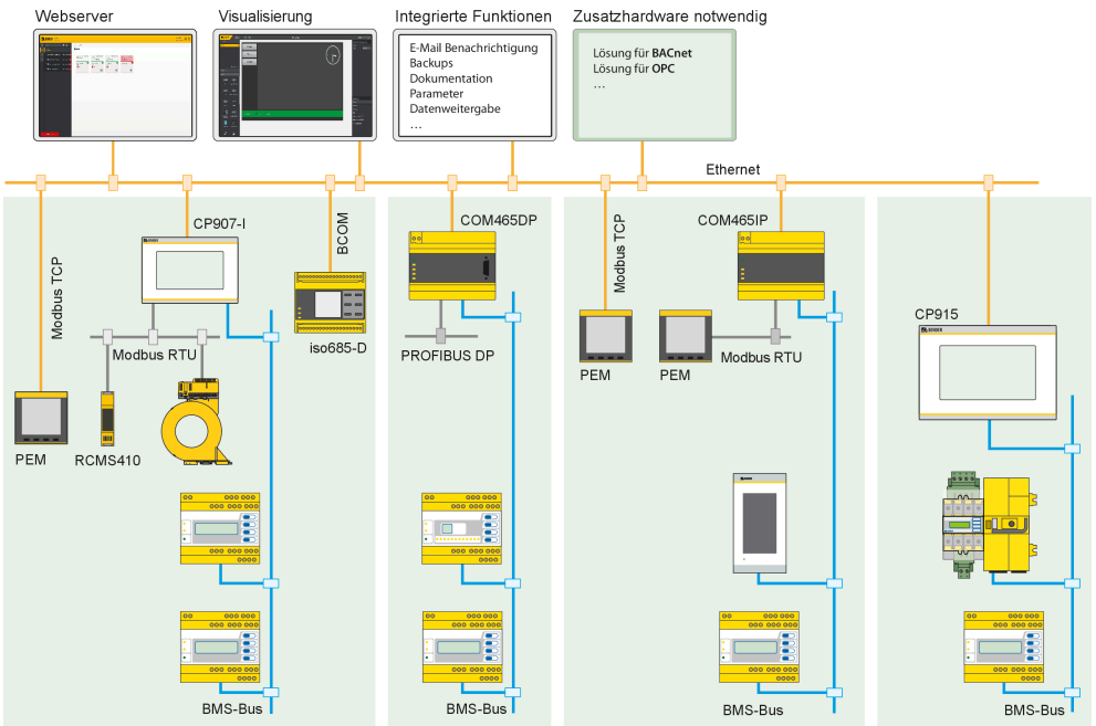
Abbildung 3-1: Systemübersicht Schnittstellen CP9...I
